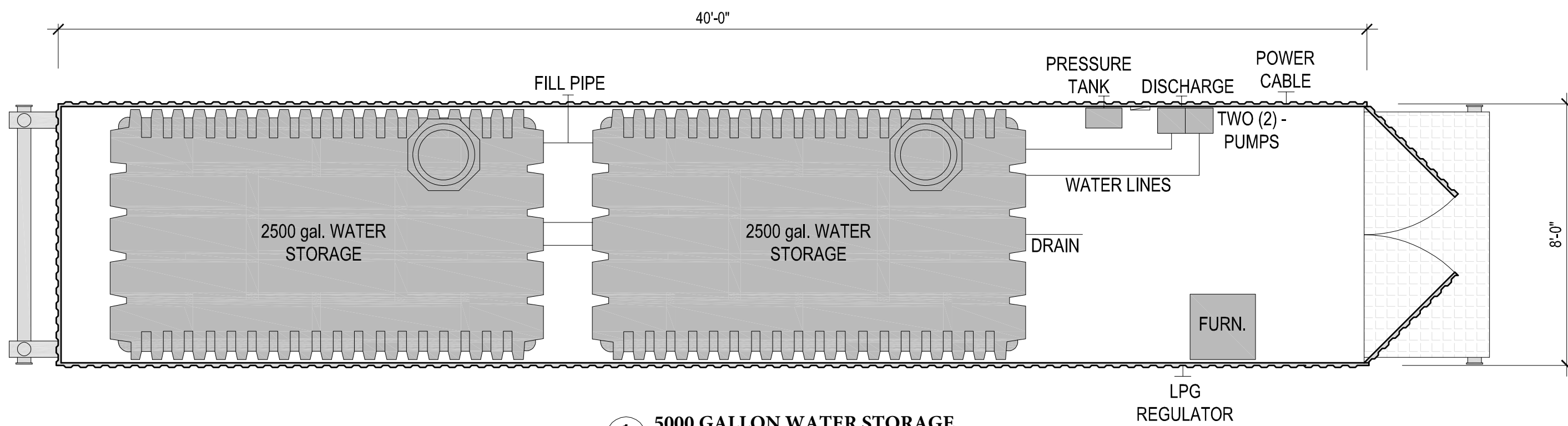
1 A-1 5000 GALLON WATER STORAGE SCALE: N.T.S.
