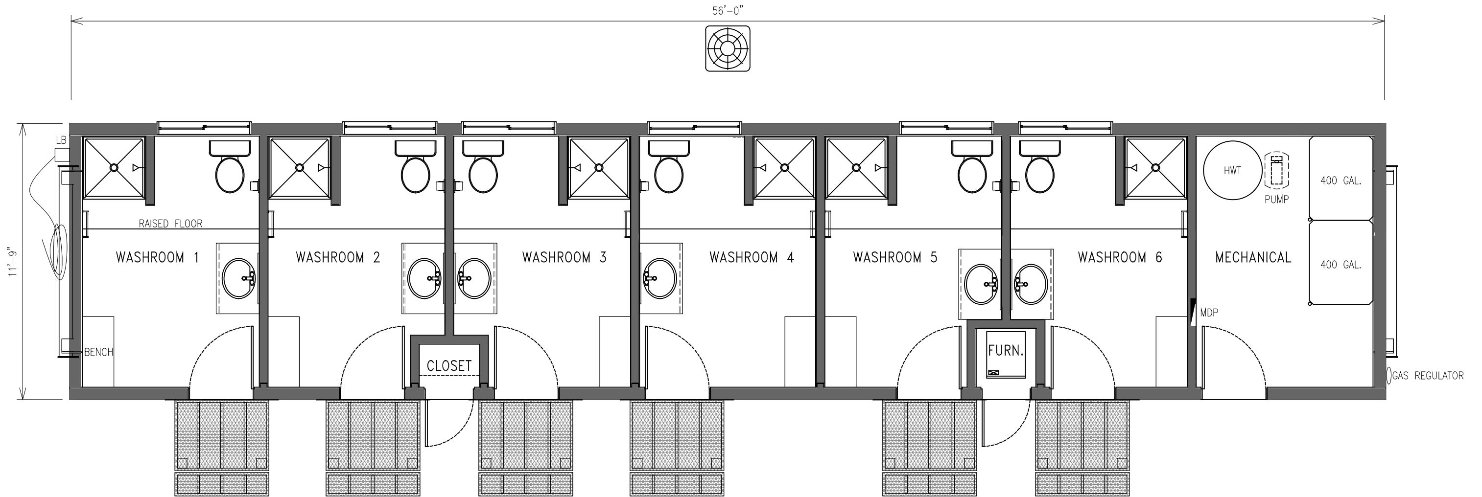
1 12'x56' WASHCAR/SOWER UNIT A-1 SCALE: N.T.S.
